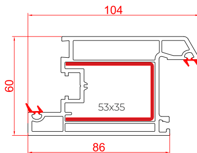
Casement Inward Door Sash RSC - 104 ID
