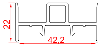
Sliding Sash Connector RSA - 22 SA
