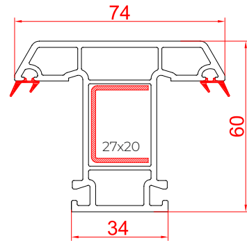
Casement T-Mullion - 74 RSC - 74 TM
