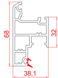
Openable Mesh RSM - 68 OM
